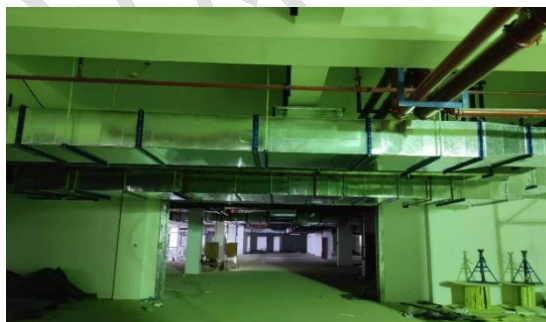
地下车库排风系统
