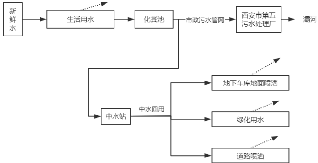
图 3-2 项目运行期水源流向图
