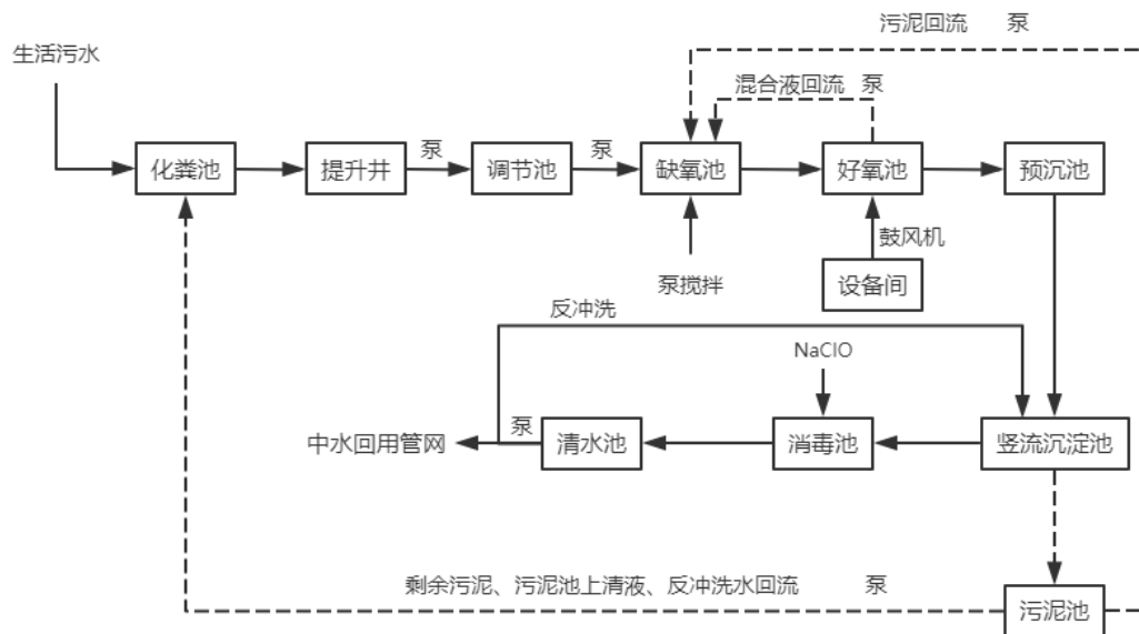
图 3-3 项目中水回用流程图
